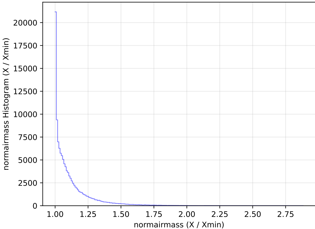
roman_v3.3_10yrs All sky u band: normairmass Histogram
