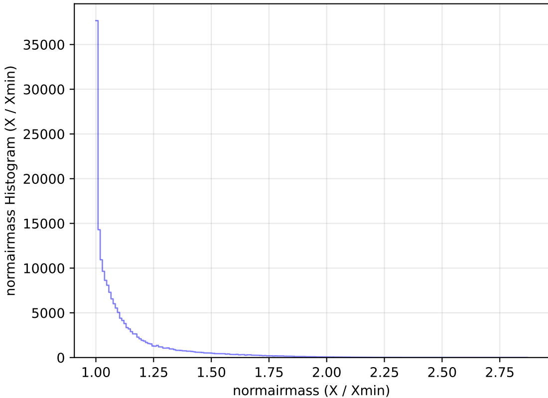
roman_v3.3_10yrs All sky g band: normairmass Histogram
