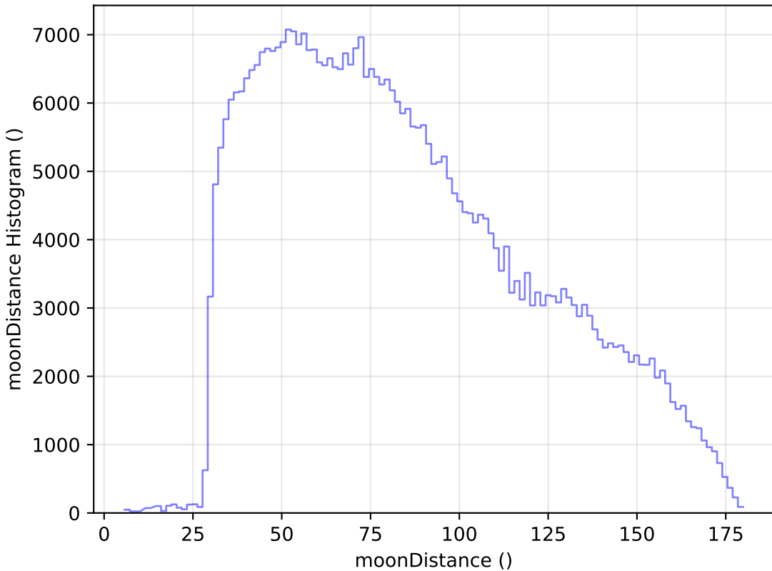
roman_v3.3_10yrs WFD z band: moonDistance Histogram
