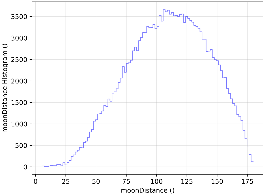
roman_v3.3_10yrs WFD g band: moonDistance Histogram
