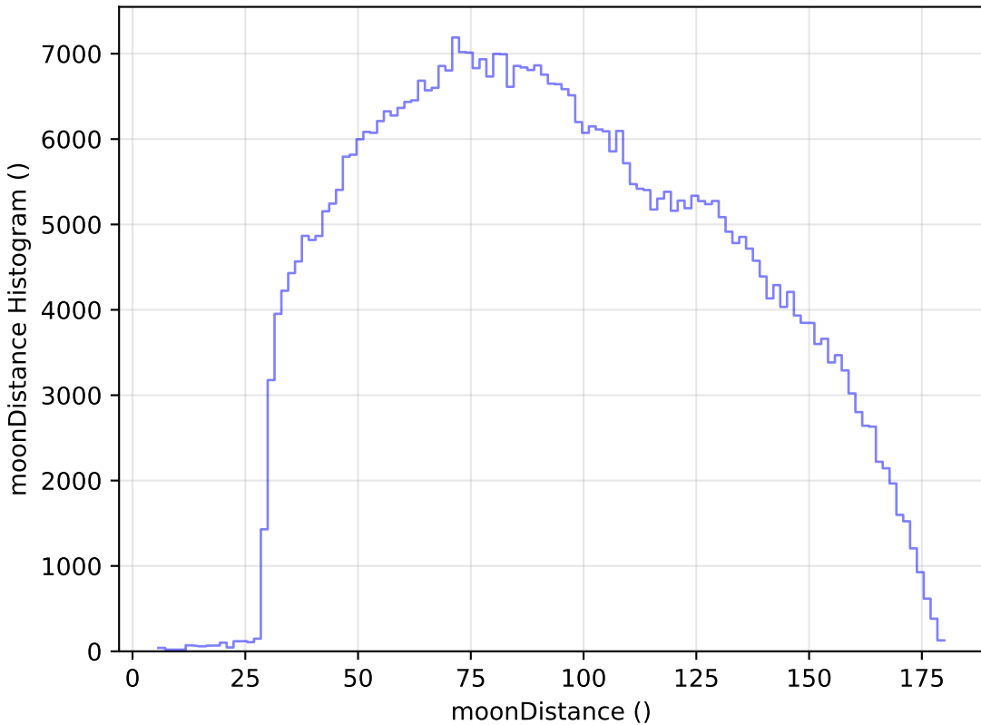
roman_v3.3_10yrs All sky i band: moonDistance Histogram
