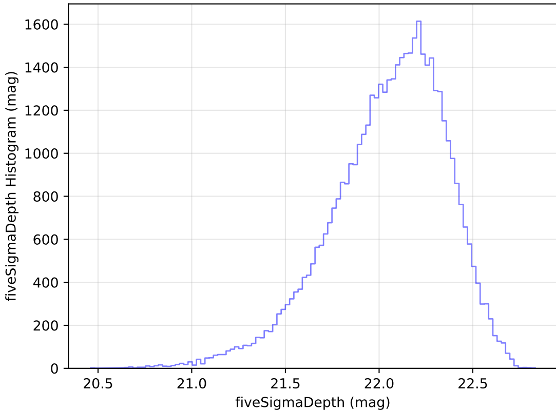
roman_v3.3_10yrs Yr 1 y band: fiveSigmaDepth Histogram
