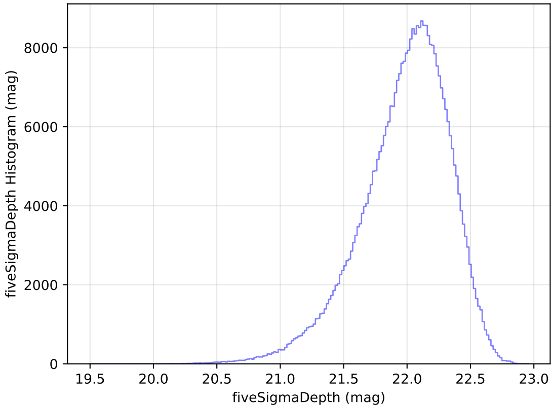
roman_v3.3_10yrs WFD y band: fiveSigmaDepth Histogram
