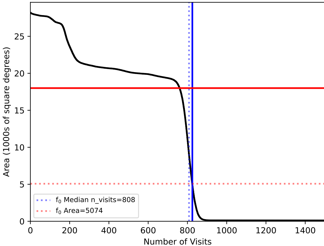
roman_v3.3_10yrs All sky: f0
