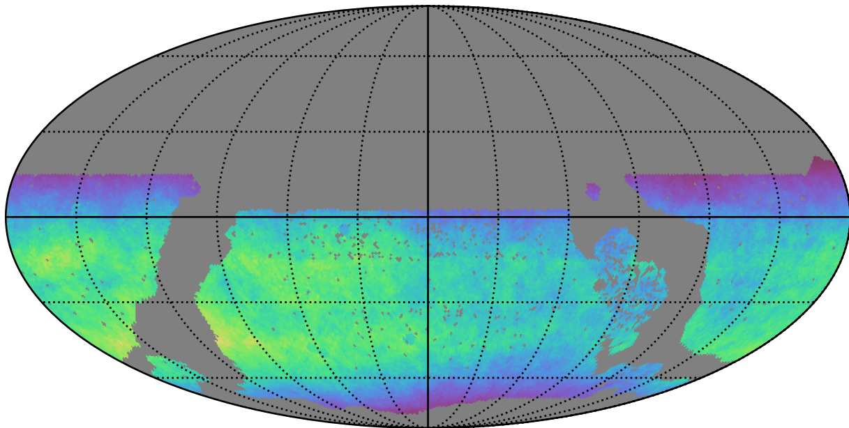
roman_v3.3_10yrs WFD y band: Normalized Teff
