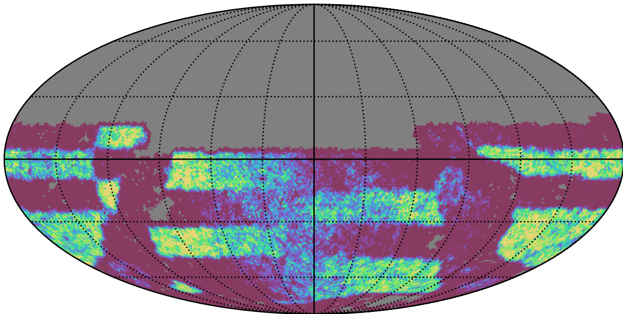
roman_v3.3_10yrs Yr 3-4 y band: NVisits
