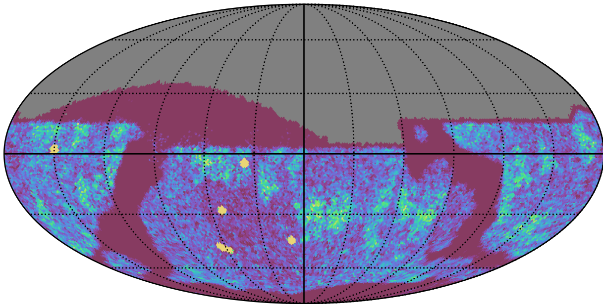
roman_v3.3_10yrs Yr 1 z band: NVisits
