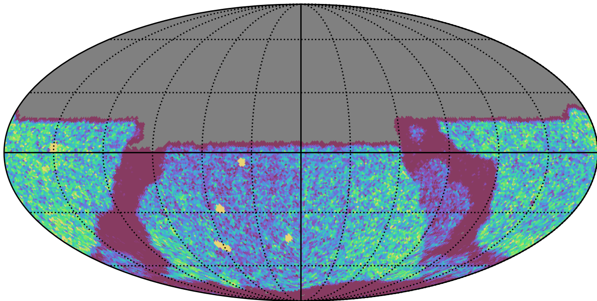
roman_v3.3_10yrs Yr 1 y band: NVisits
