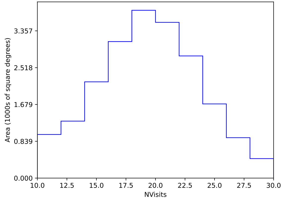
roman_v3.3_10yrs Yr 1 y band: NVisits
