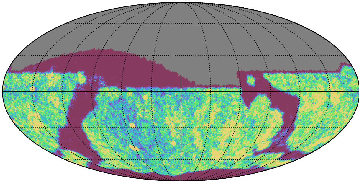
roman_v3.3_10yrs Yr 1 i band: NVisits
