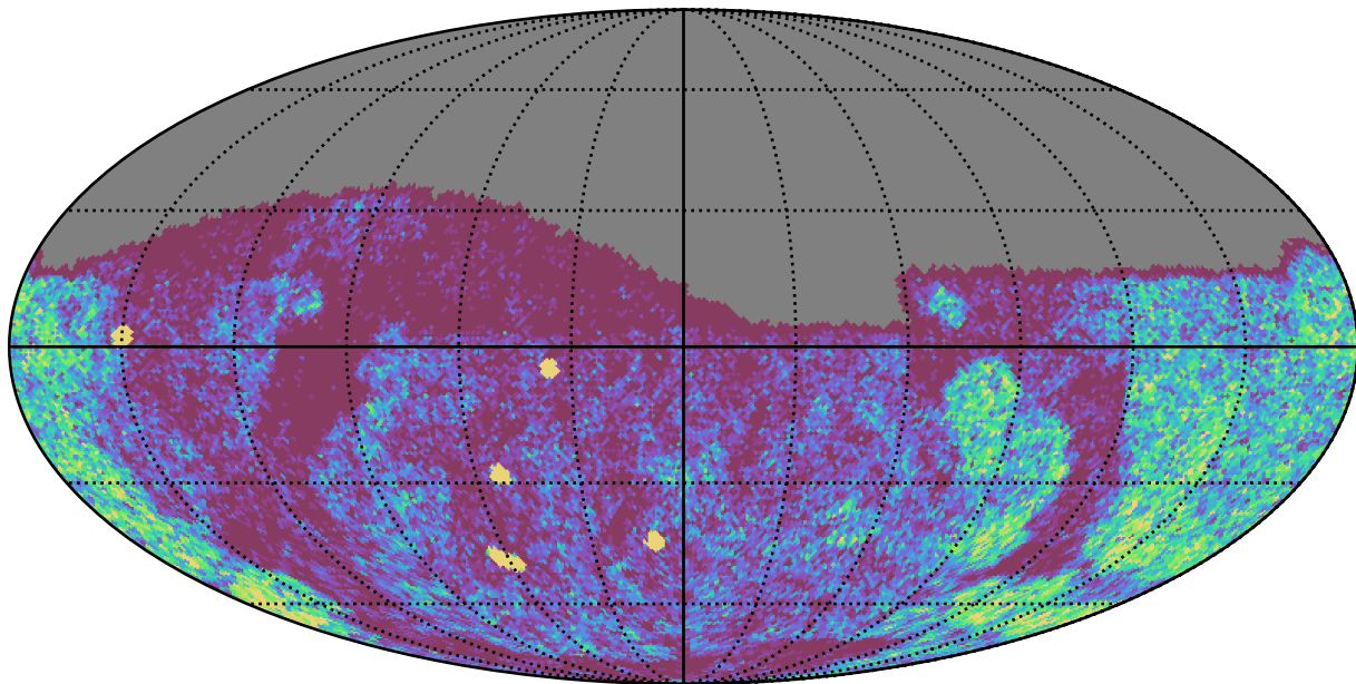
roman_v3.3_10yrs Yr 1 g band: NVisits
