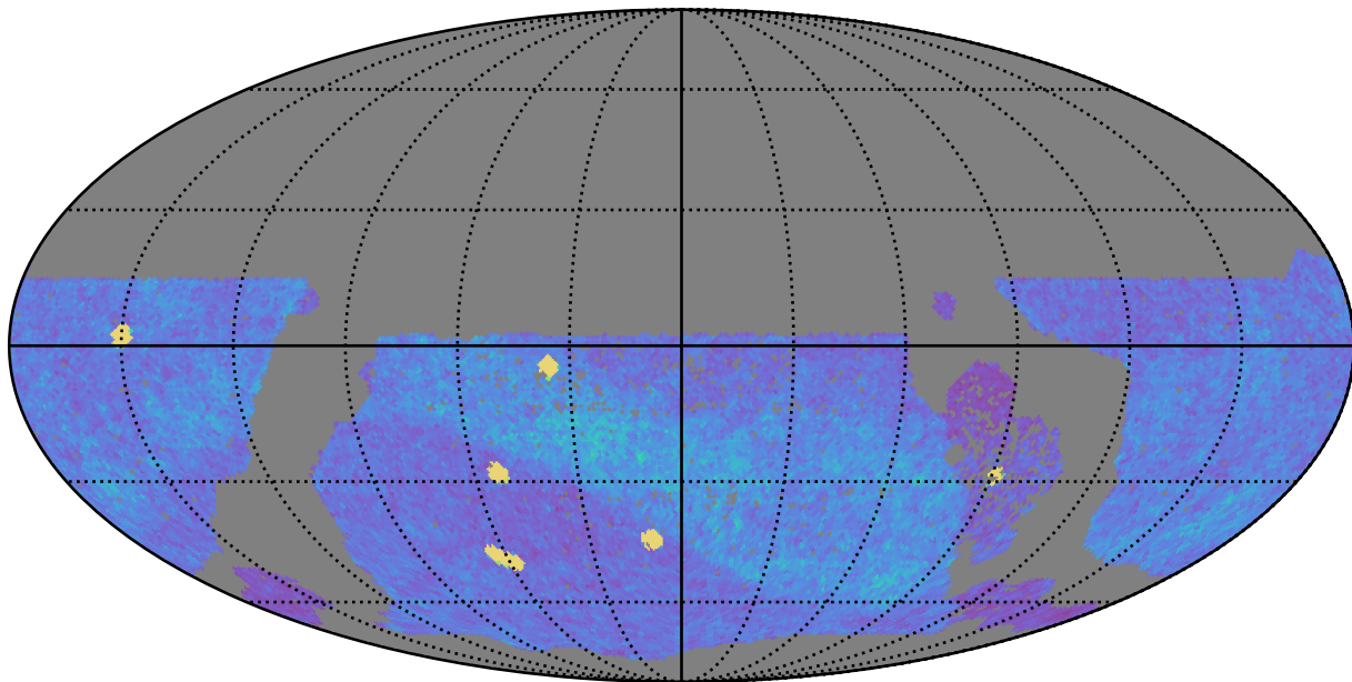
roman_v3.3_10yrs WFD z band: NVisits
