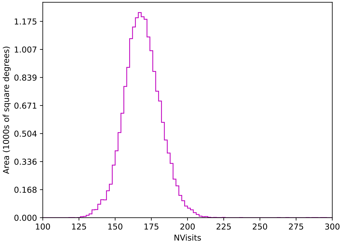
roman_v3.3_10yrs WFD z band: NVisits
