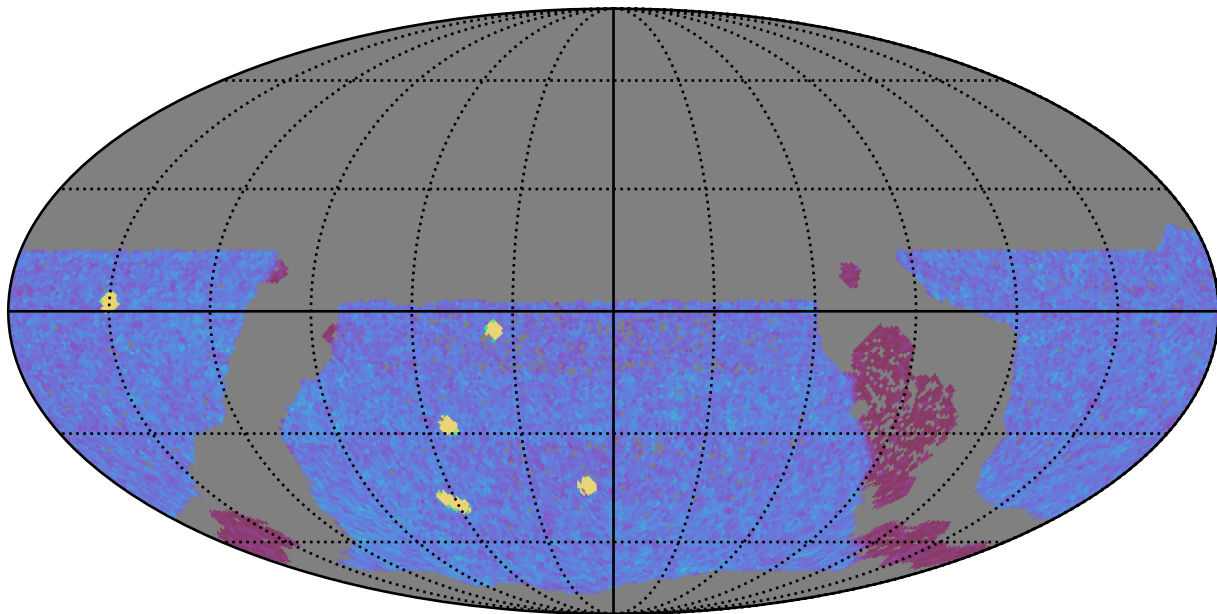
roman_v3.3_10yrs WFD y band: NVisits
