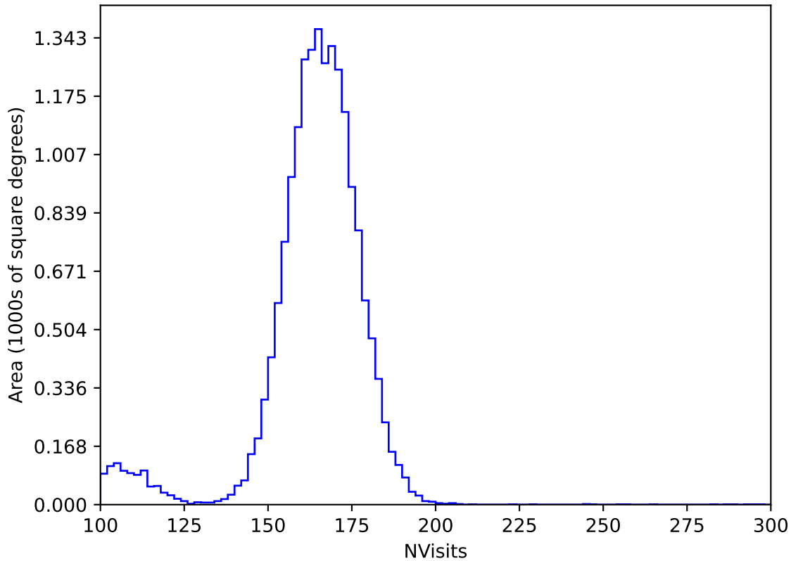
roman_v3.3_10yrs WFD y band: NVisits
