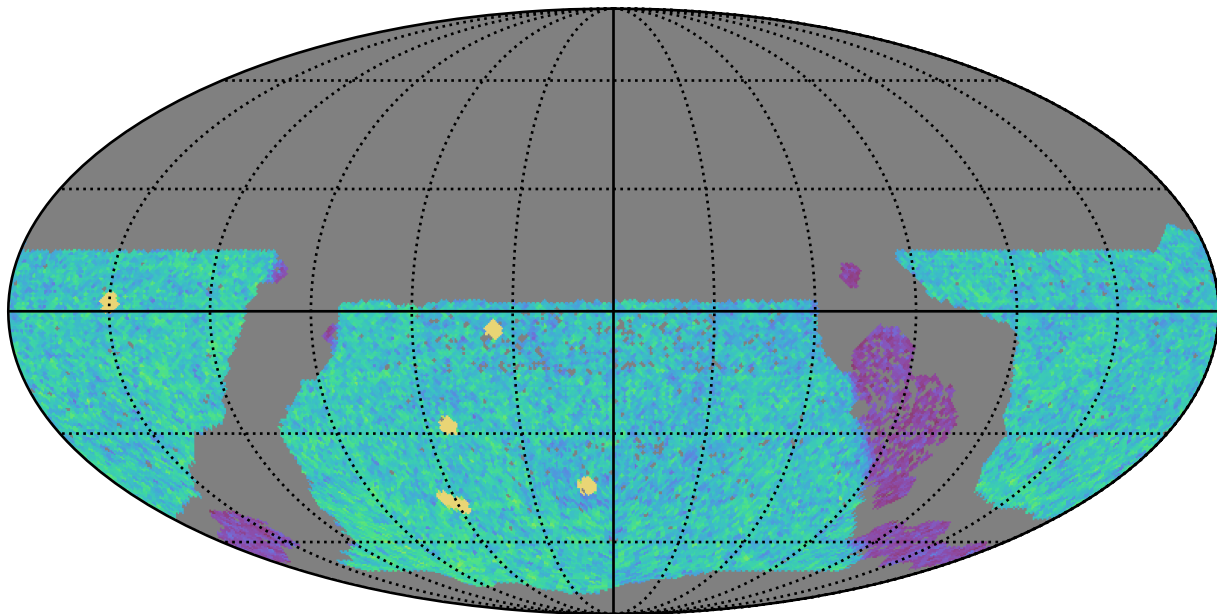
roman_v3.3_10yrs WFD u band: NVisits
