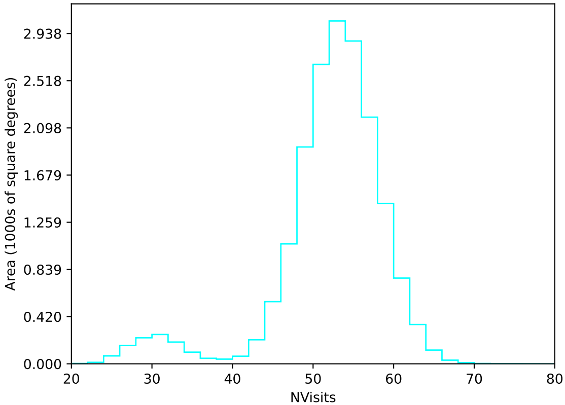
roman_v3.3_10yrs WFD u band: NVisits
