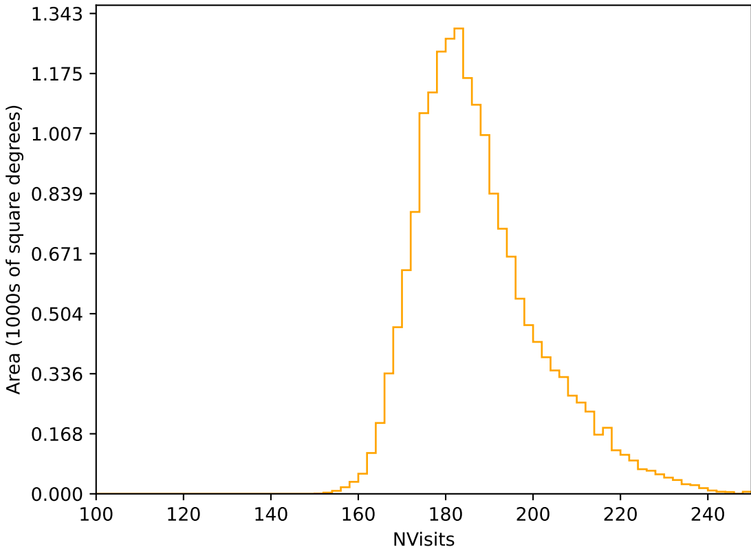
roman_v3.3_10yrs WFD r band: NVisits
