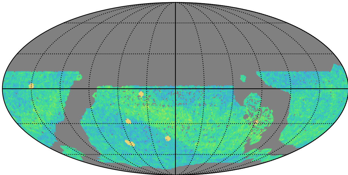
roman_v3.3_10yrs WFD i band: NVisits
