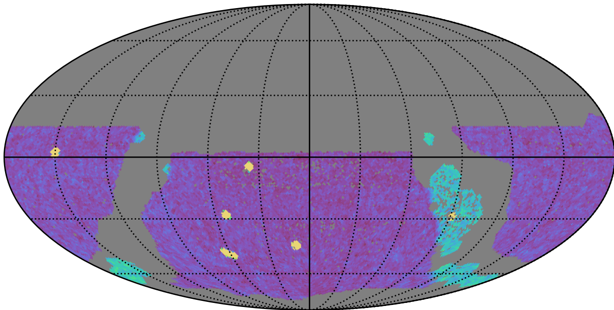
roman_v3.3_10yrs WFD g band: NVisits
