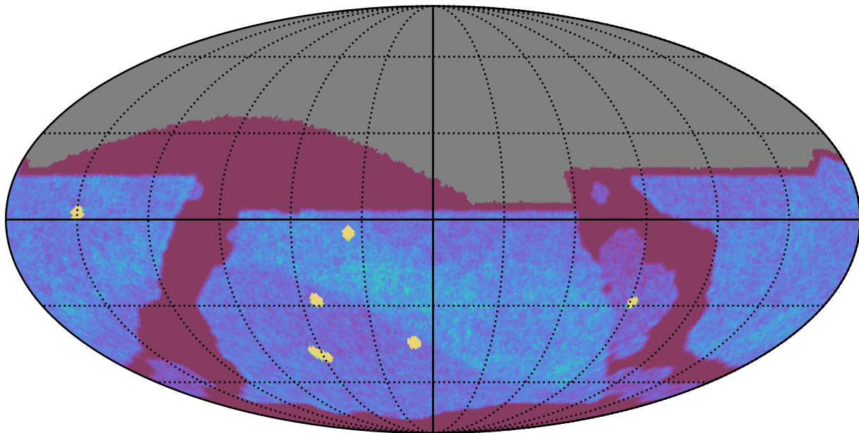
roman_v3.3_10yrs All sky z band: NVisits
