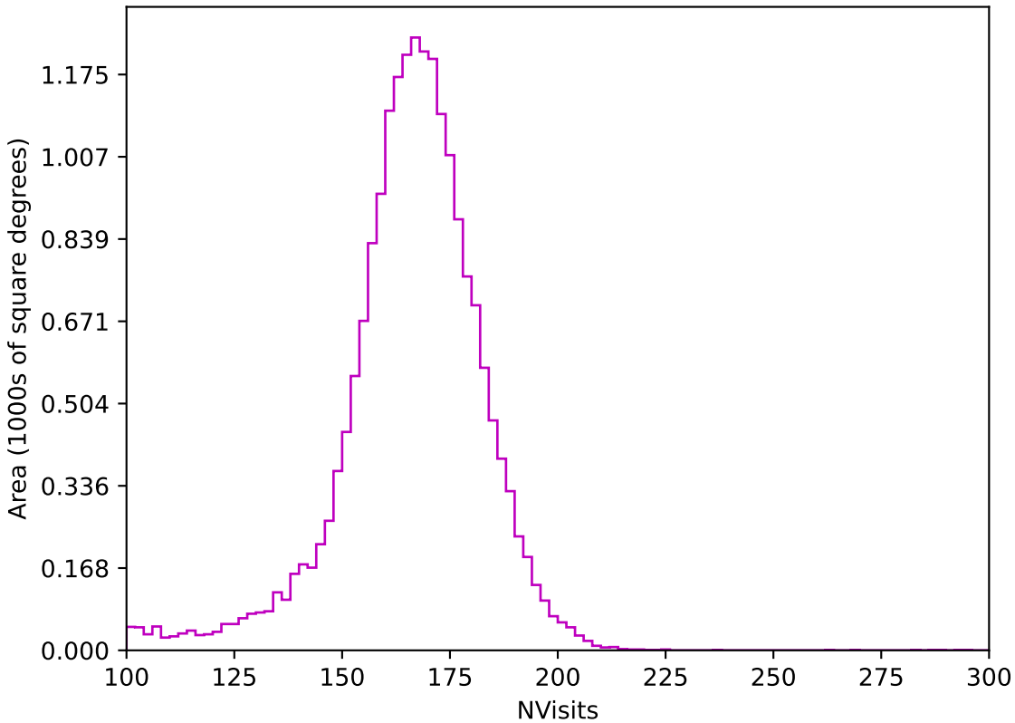
roman_v3.3_10yrs All sky z band: NVisits
