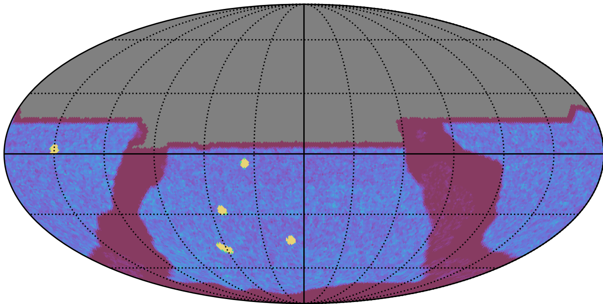
roman_v3.3_10yrs All sky y band: NVisits
