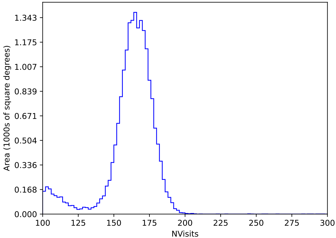
roman_v3.3_10yrs All sky y band: NVisits
