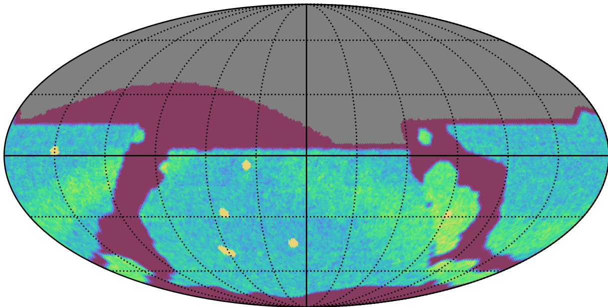
roman_v3.3_10yrs All sky r band: NVisits
