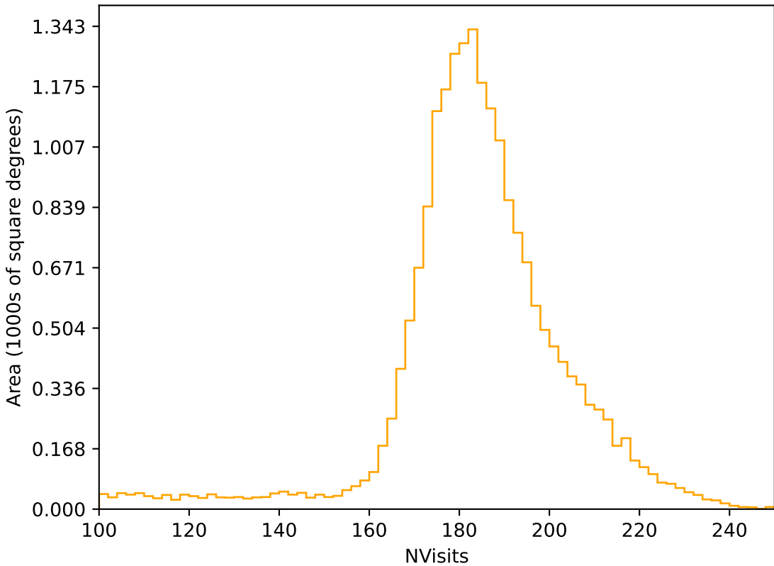
roman_v3.3_10yrs All sky r band: NVisits
