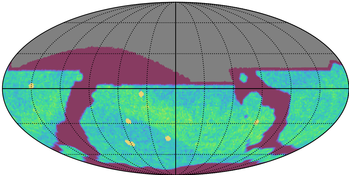
roman_v3.3_10yrs All sky i band: NVisits
