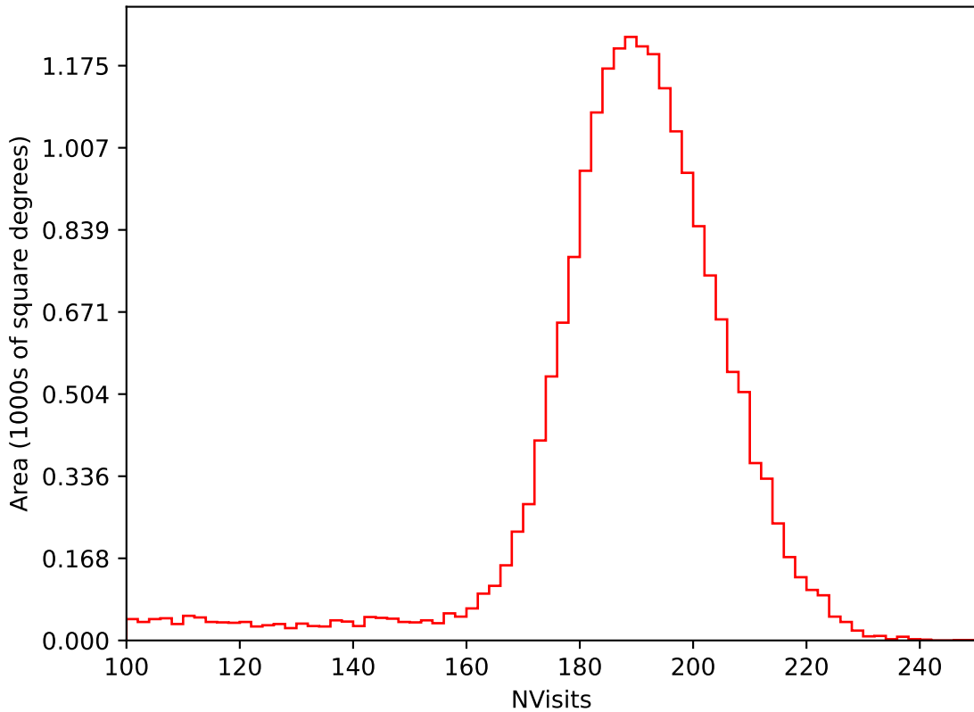
roman_v3.3_10yrs All sky i band: NVisits
