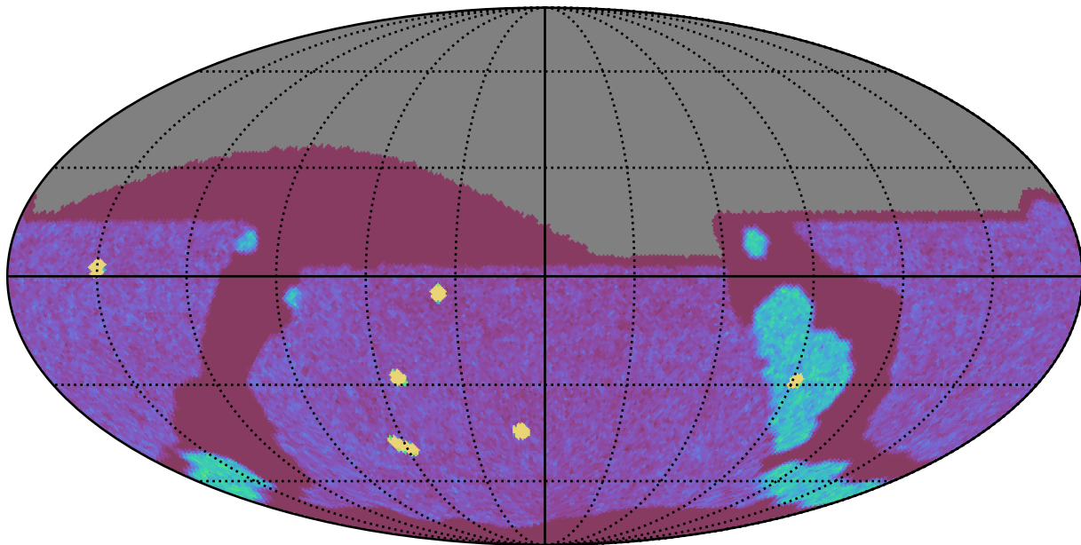
roman_v3.3_10yrs All sky g band: NVisits
