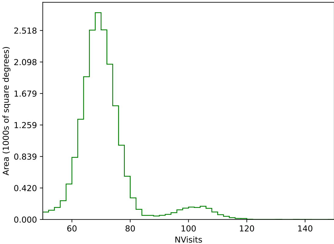
roman_v3.3_10yrs All sky g band: NVisits
