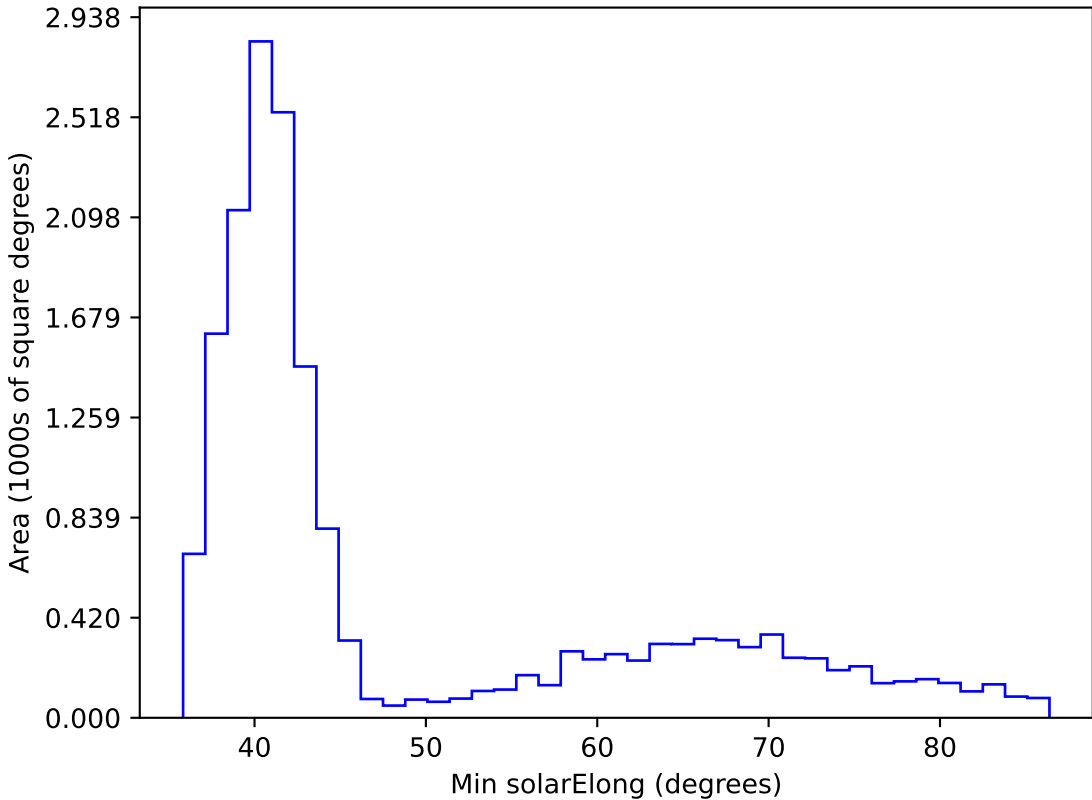
roman_v3.3_10yrs WFD z band: Min solarElong
