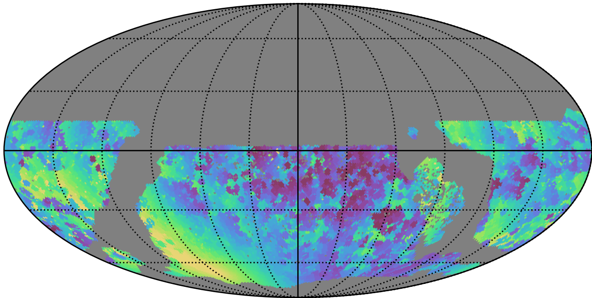
roman_v3.3_10yrs WFD y band: Min solarElong
