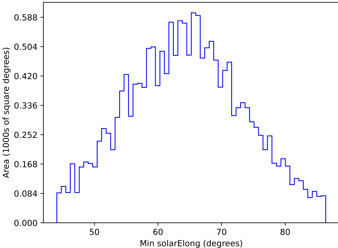
roman_v3.3_10yrs WFD y band: Min solarElong
