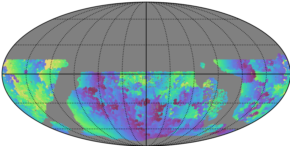
roman_v3.3_10yrs WFD u band: Min solarElong
