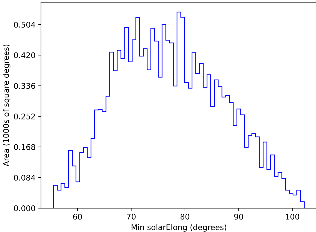
roman_v3.3_10yrs WFD u band: Min solarElong
