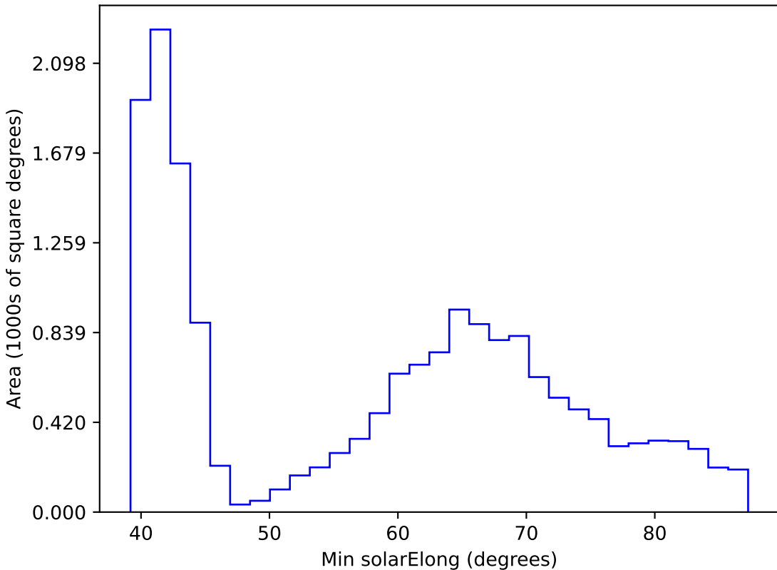
roman_v3.3_10yrs WFD r band: Min solarElong
