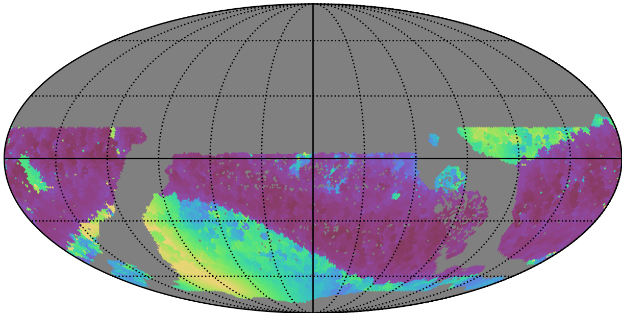
roman_v3.3_10yrs WFD i band: Min solarElong
