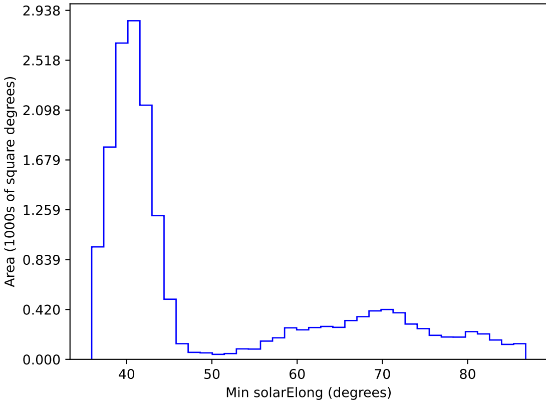
roman_v3.3_10yrs WFD i band: Min solarElong
