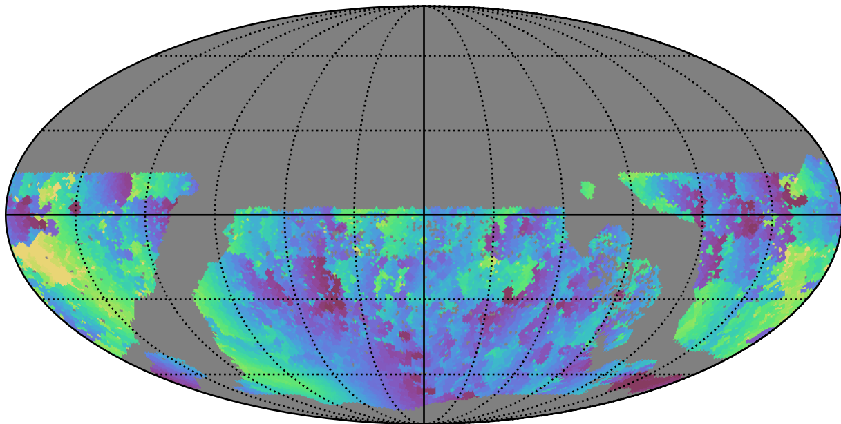
roman_v3.3_10yrs WFD g band: Min solarElong
