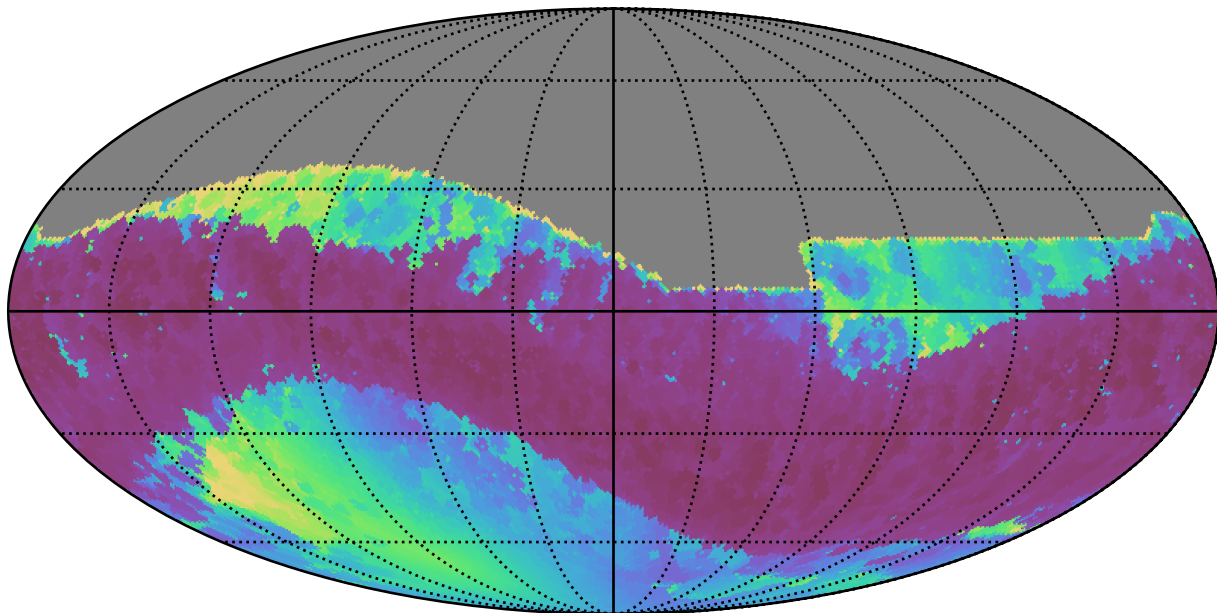
roman_v3.3_10yrs All sky z band: Min solarElong
