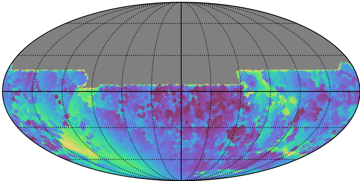
roman_v3.3_10yrs All sky y band: Min solarElong
