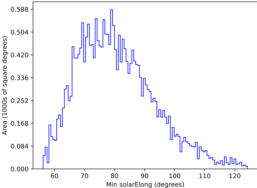
roman_v3.3_10yrs All sky u band: Min solarElong
