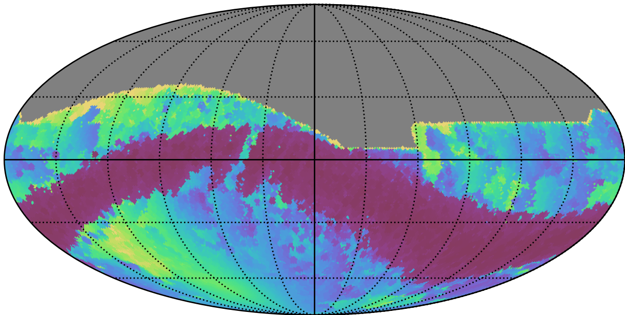
roman_v3.3_10yrs All sky r band: Min solarElong
