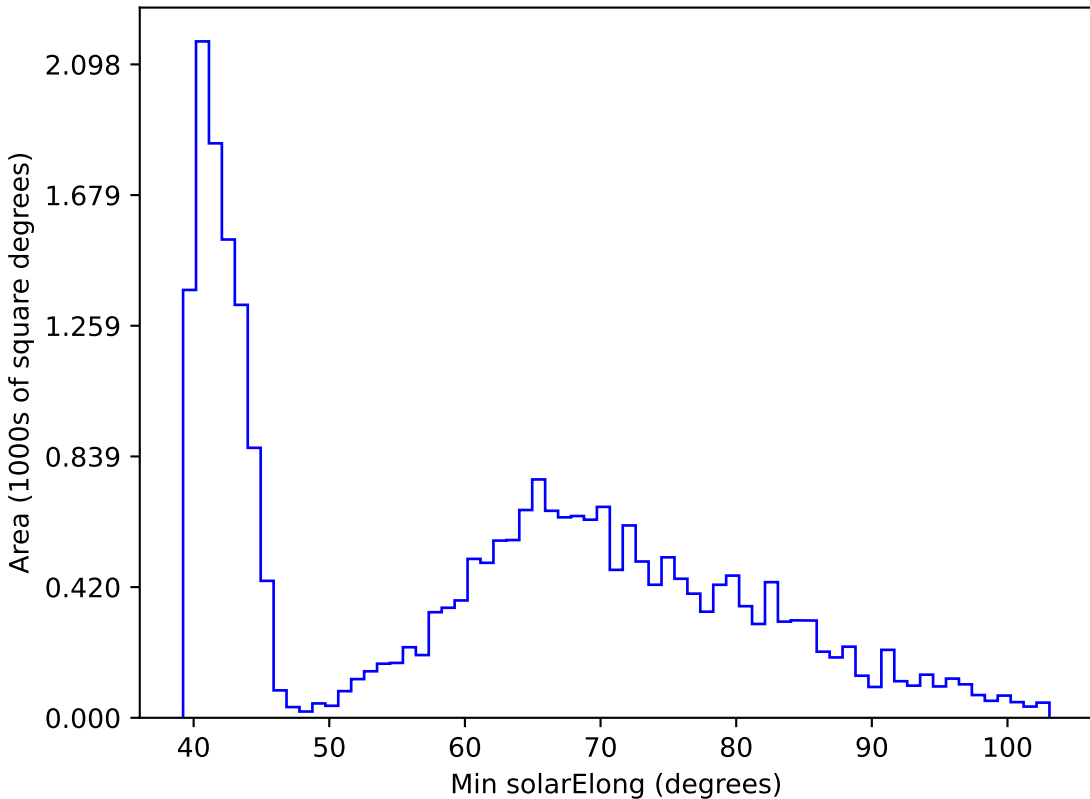
roman_v3.3_10yrs All sky r band: Min solarElong
