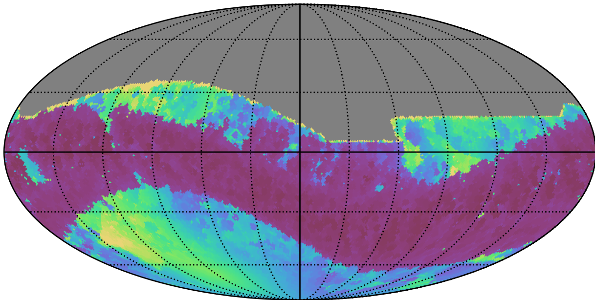
roman_v3.3_10yrs All sky i band: Min solarElong
