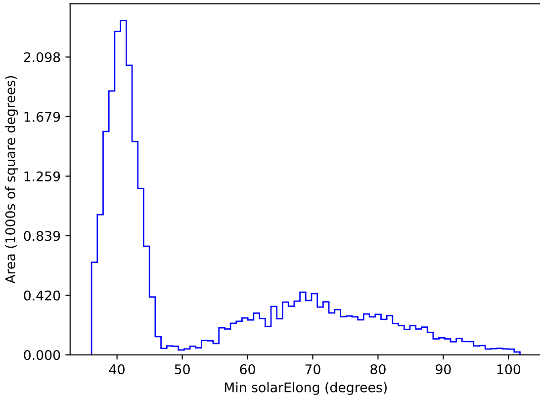
roman_v3.3_10yrs All sky i band: Min solarElong
